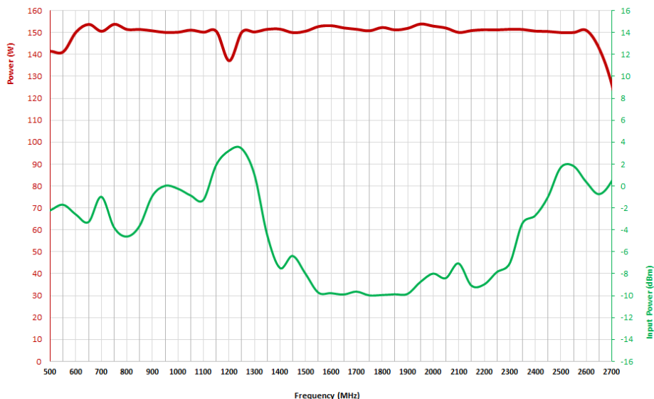
VM2K Input & Power
